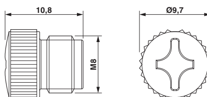
Maßzeichnung
