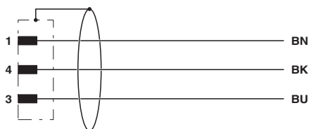
Kontaktbelegung der M12-Stecker
