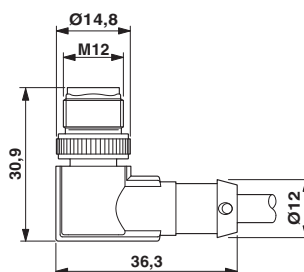
Stecker M12 x 1, gewinkelt, geschirmt
