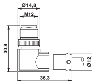
Maßzeichnung
