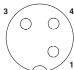
Polbild Buchse M12, 3-polig, A-kodiert, Ansicht Buchsenseite
