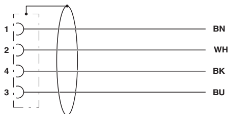
Kontaktbelegung der M12-Buchse
