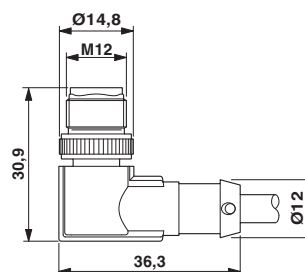
Stecker M12 x 1, gewinkelt, geschirmt
