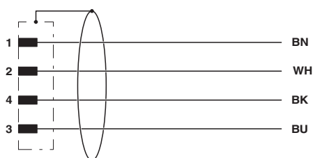
Kontaktbelegung des M12-Steckers
