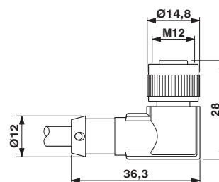
Buchse M12 x 1, gewinkelt, geschirmt
