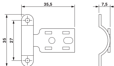
Maßzeichnung
