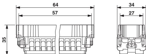
Maßzeichnung
