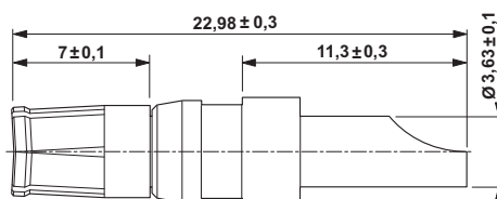
Maßzeichnung
