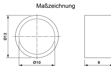
Schraubendruckmutter
