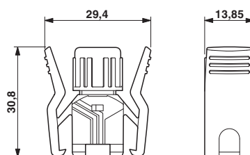
Maßzeichnung
