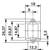
Maßzeichnung
