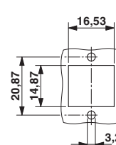
Maßzeichnung
