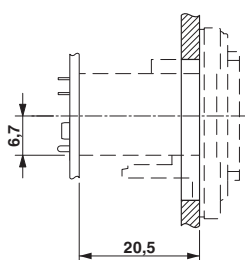
Maßzeichnung
