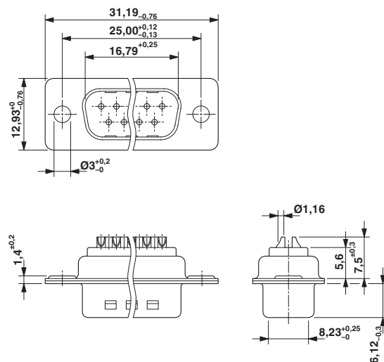
Maßzeichnung
