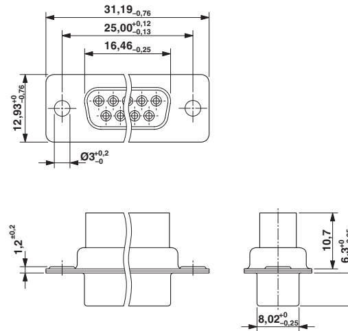
Maßzeichnung
