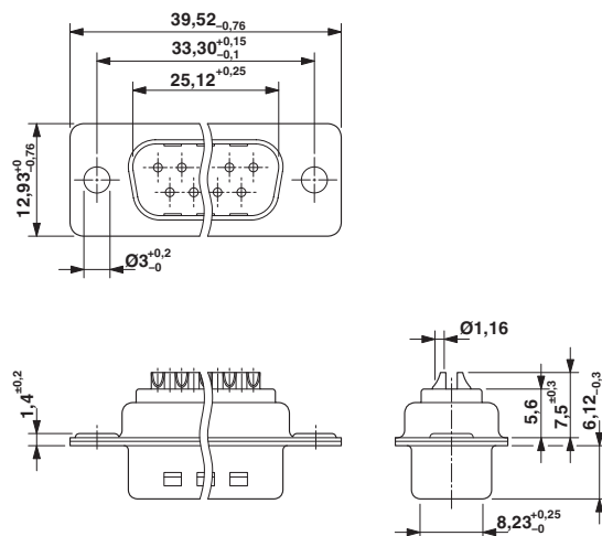
Maßzeichnung
