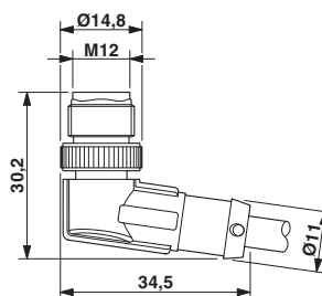
Maßzeichnung
