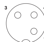
Polbild Buchse M12, 3-polig, A-kodiert, Ansicht Buchsen-seite
