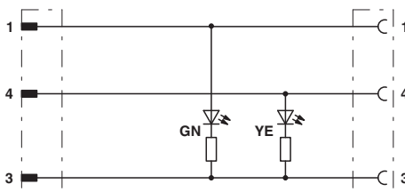
Schaltplan
