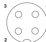
Polbild Buchse M12, 12-polig, A-kodiert, Ansicht Buchsenseite
