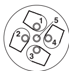
Kabelanschlussseite M12 (Schraubanschluss)
