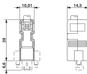
Maßzeichnung
