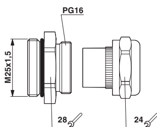
Maßzeichnung
