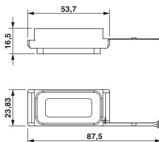
Maßzeichnung
