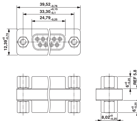
Maßzeichnung
