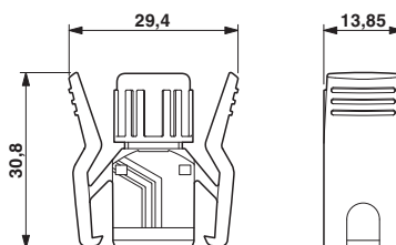
Maßzeichnung
