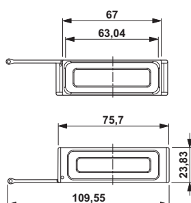
Maßzeichnung
