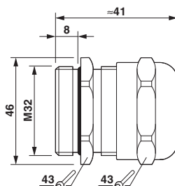
Maßzeichnung
