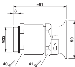
Maßzeichnung
