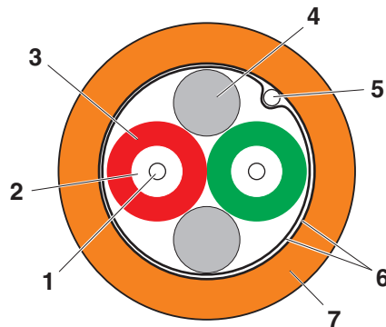
Schemazeichnung
