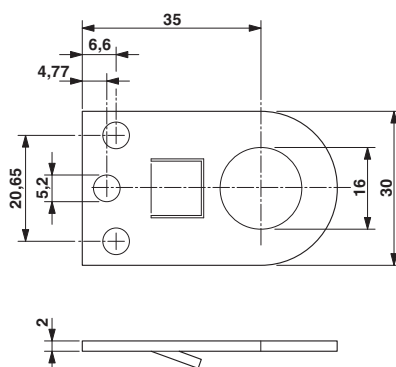
Maßzeichnung
