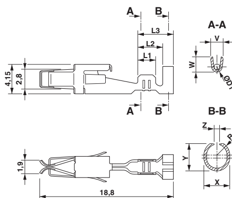
Maßzeichnung
