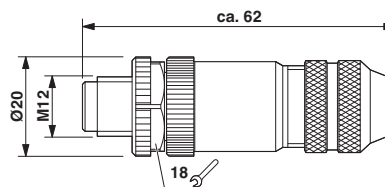
Maßzeichnung
