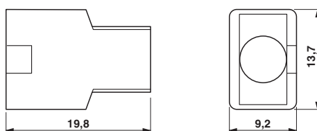
Maßzeichnung
