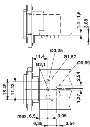
Maßzeichnung
