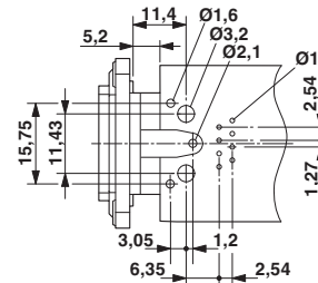
Bohrplan
