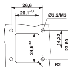
Maßzeichnung
