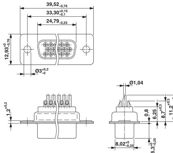
Maßzeichnung
