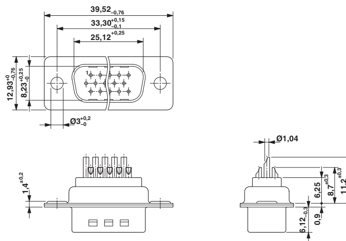
Maßzeichnung
