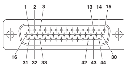
Schemazeichnung
