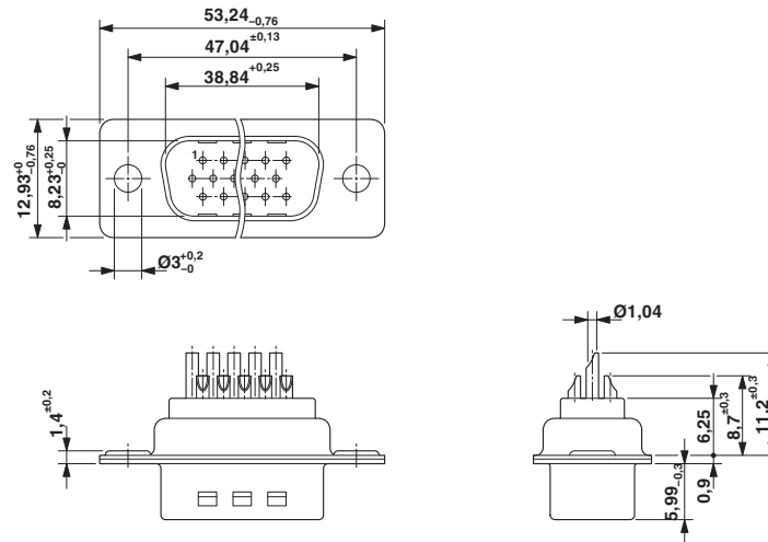
Maßzeichnung
