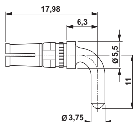
Maßzeichnung
