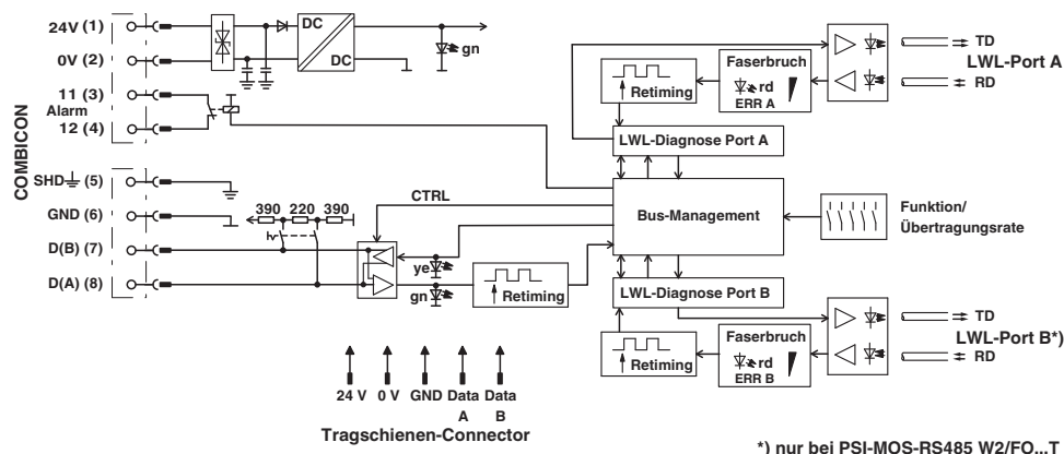
Blockschaltbild
