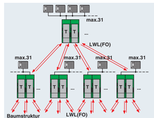
Redundante Sternstruktur
