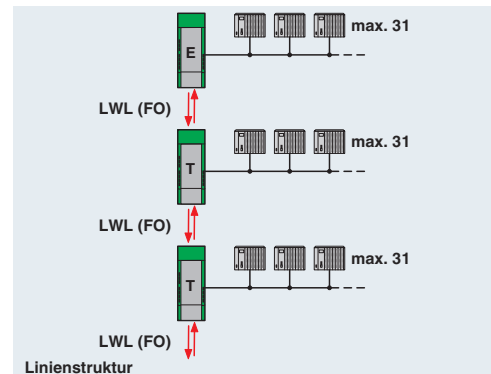
Applikationszeichnung
