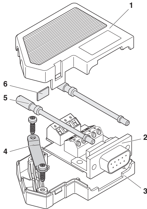
Schemazeichnung
