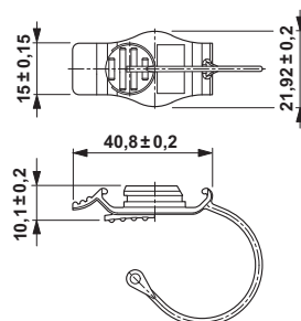
Maßzeichnung
