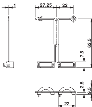
Maßzeichnung
