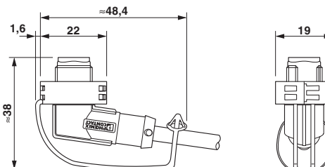
Maßzeichnung
