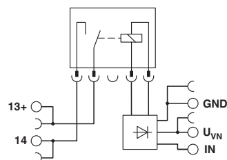
Schaltplan
