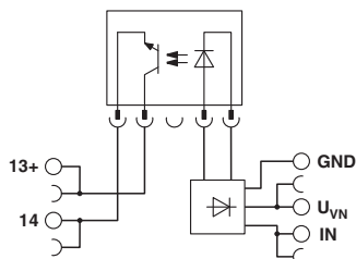
Schaltplan
