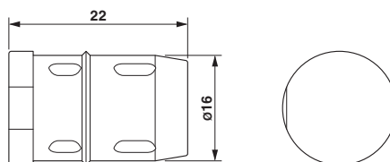
Maßzeichnung
