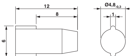
Maßzeichnung
