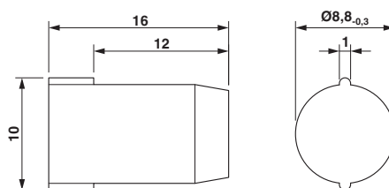
Maßzeichnung
