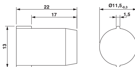
Maßzeichnung
