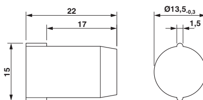
Maßzeichnung
