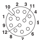
Polbild Buchse M12, 12-polig, Ansicht Buchsenseite
